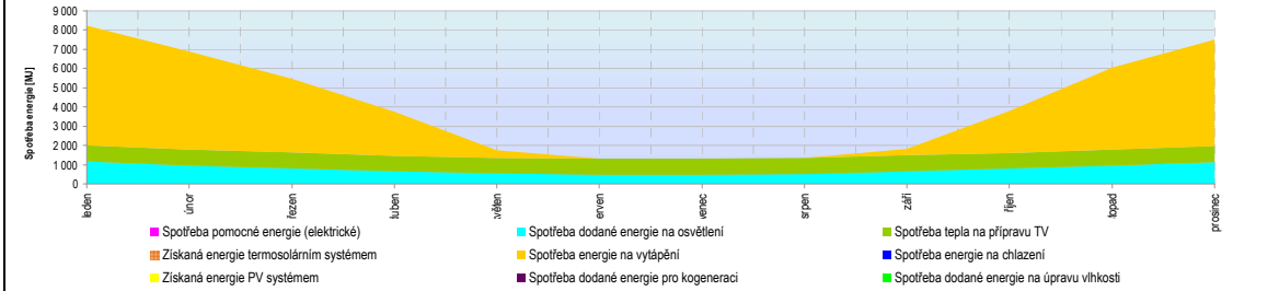
Celková roční dodaná energie do budovy s vlivem systému využívající OZE a kogenerace [MJ]
