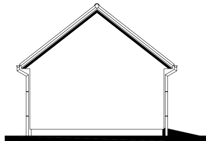
POHLED BOČNÍ
