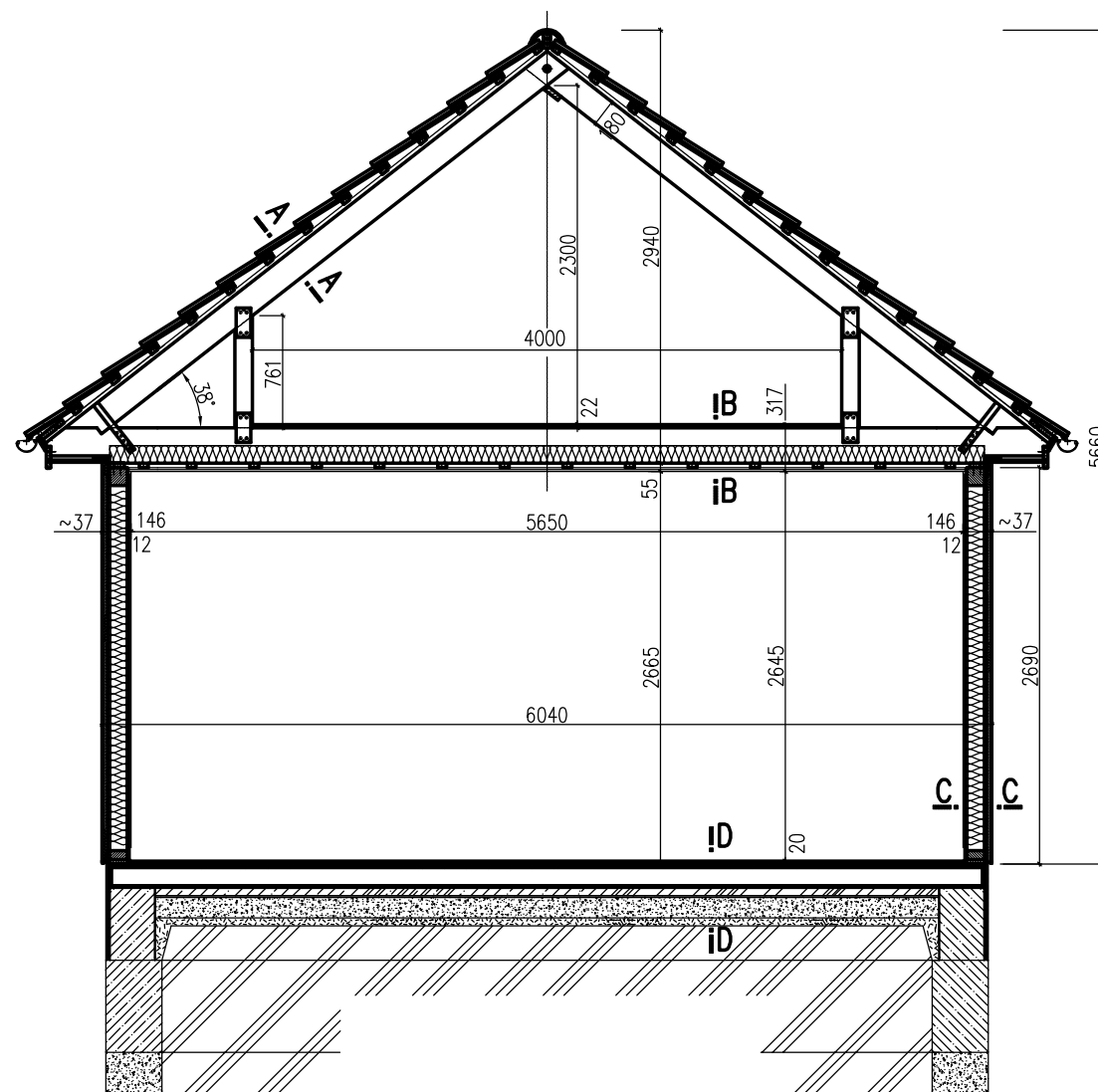
ŘEZ GARÁŽÍ
