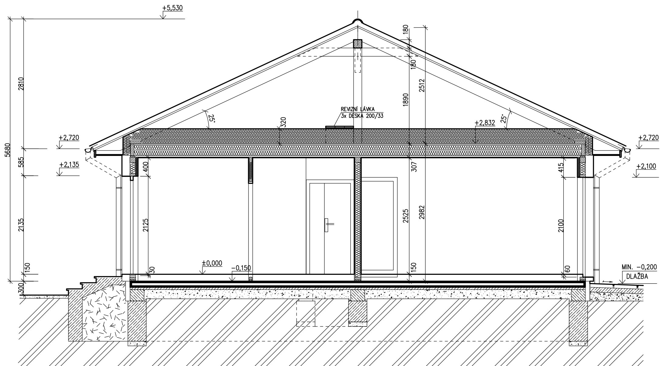
SPODNÍ STAVBA ŘEŠENA V SAMOSTATNÉ ČÁSTI DOKUMENTACE PROJEKTANTEM ODBĚRATELE
